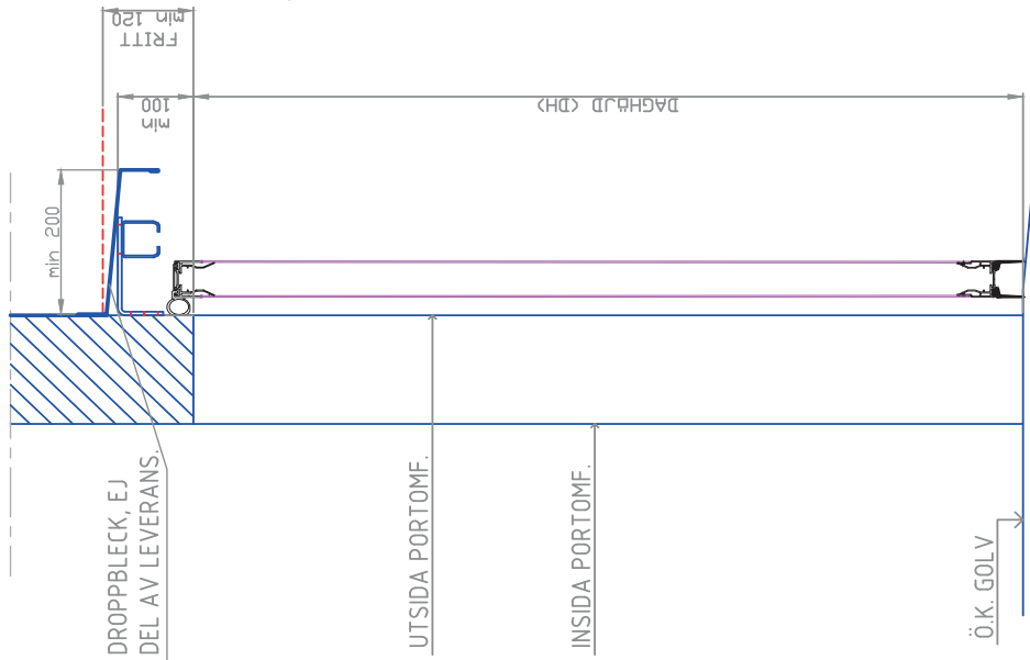
VERTIKALSEKTION 1:10
